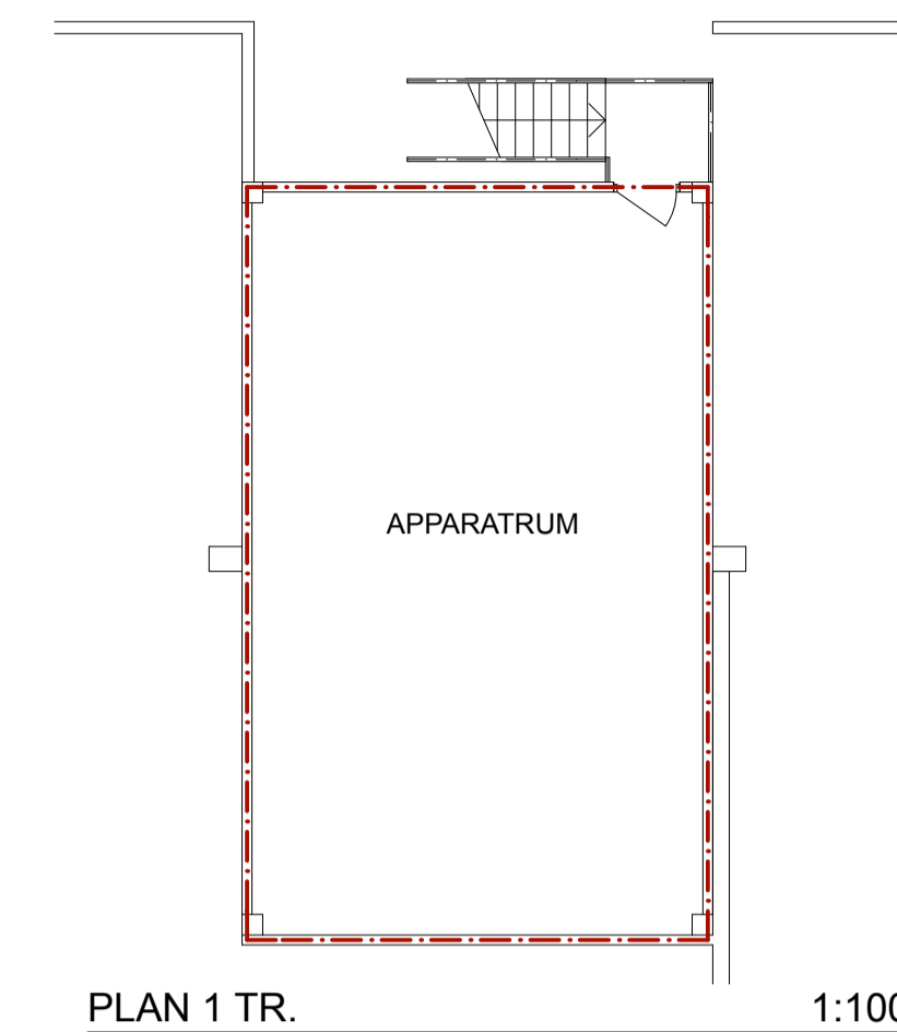
PLAN 1 TR. 1:100
